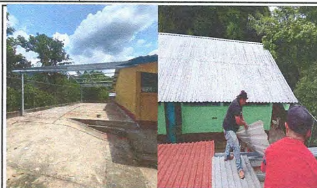
Foto 2: Mejora de techo de lámina troquelada cal. 26 en portico de Ingreso, entre 2 aulas laterales y área del fondo con un 70 % de avance
